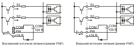
Рисунок 3-13 Режим PNP
