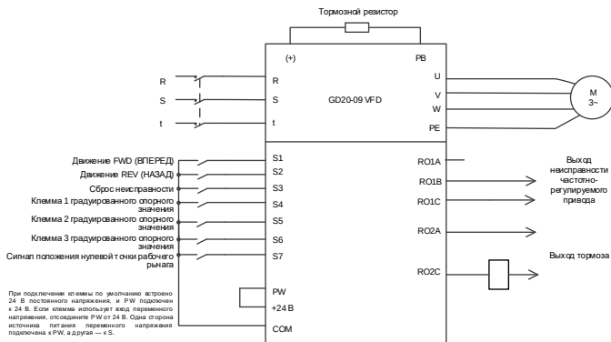
Рисунок 4-6 Подключение рабочего рычага с градуированным опорным значением
