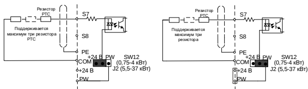
Рисунок 3-15 Подключение PTC
