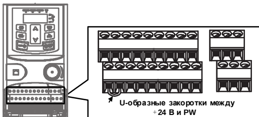
Рисунок 3-11 U-образная закоротка
